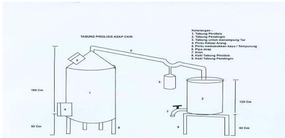
Gambar I E. 1 Contoh Alat Pembuat Asap Cair
