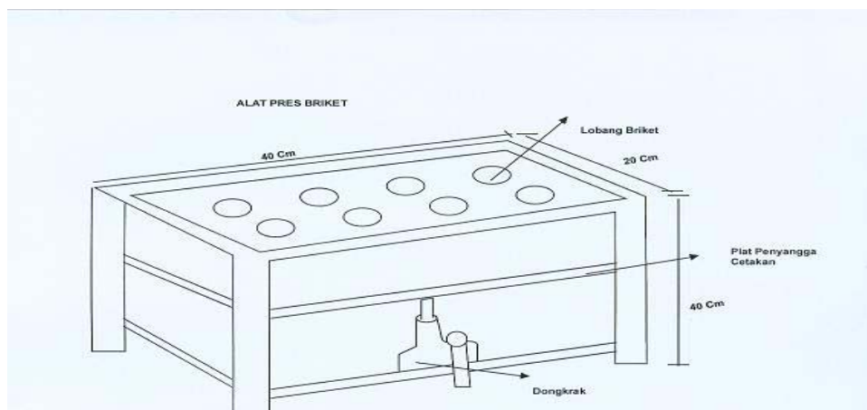
Gambar I E. 2 Contoh Alat Pembuat Briket Arang
